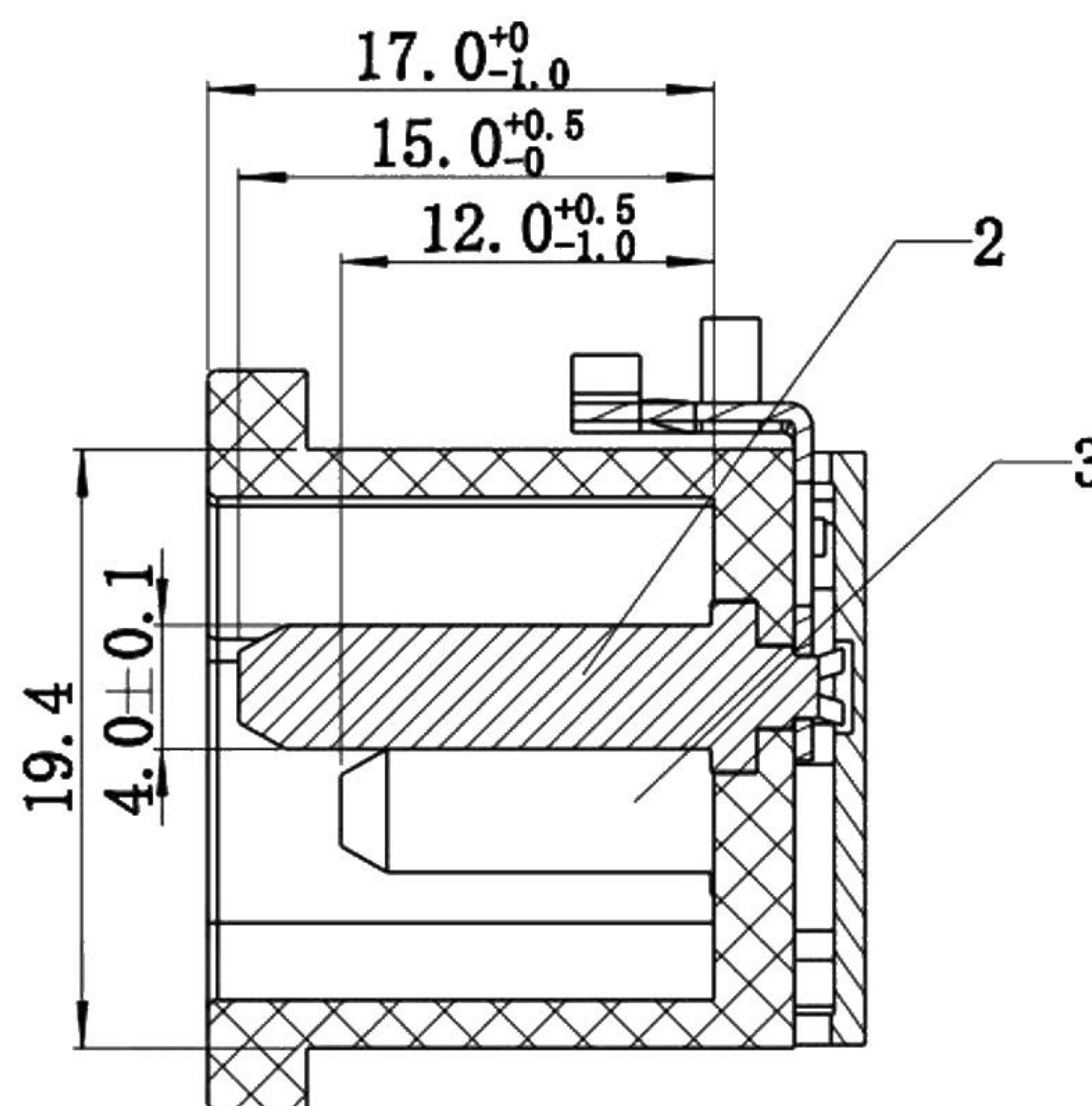
剖面 A-A
