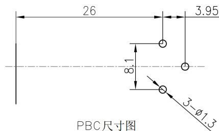
PBC尺寸图
