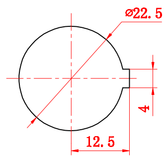
安装尺寸
