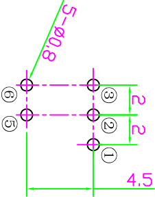
P.C.B 设计参考尺寸
