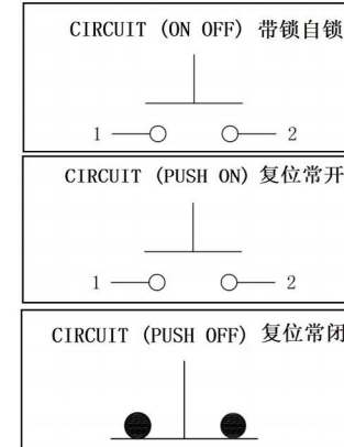
电气原理图
