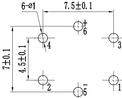
元件面孔位图
