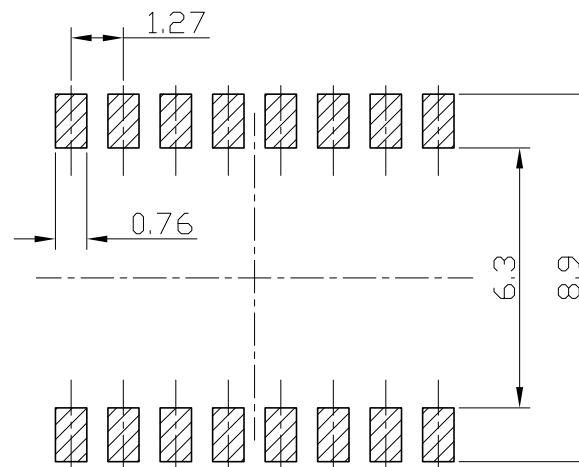
P.C.B LAYOUT
