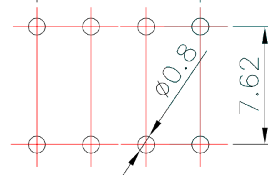
PCB Layout(Pattern Side)
