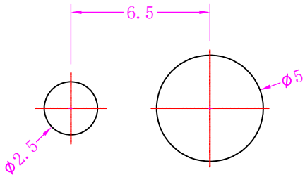
安装孔尺寸
