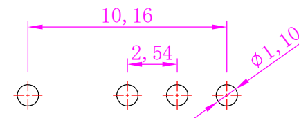
安装孔尺寸
