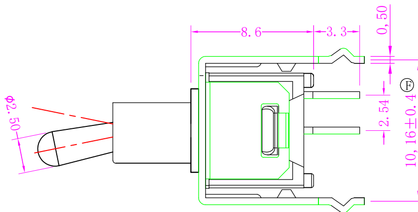
标注: ①-⑦ 尺寸的重点检验尺寸
