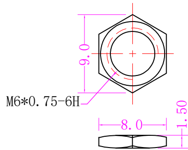
六角螺母
