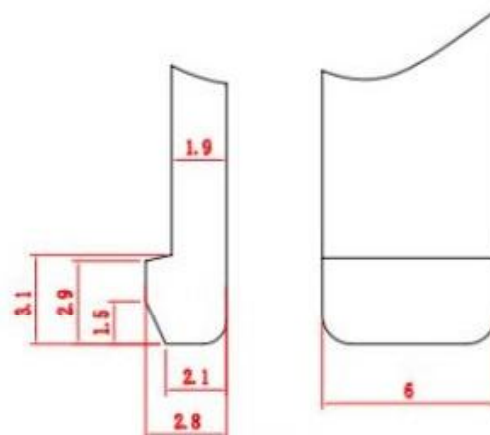
锁舌参考规格
