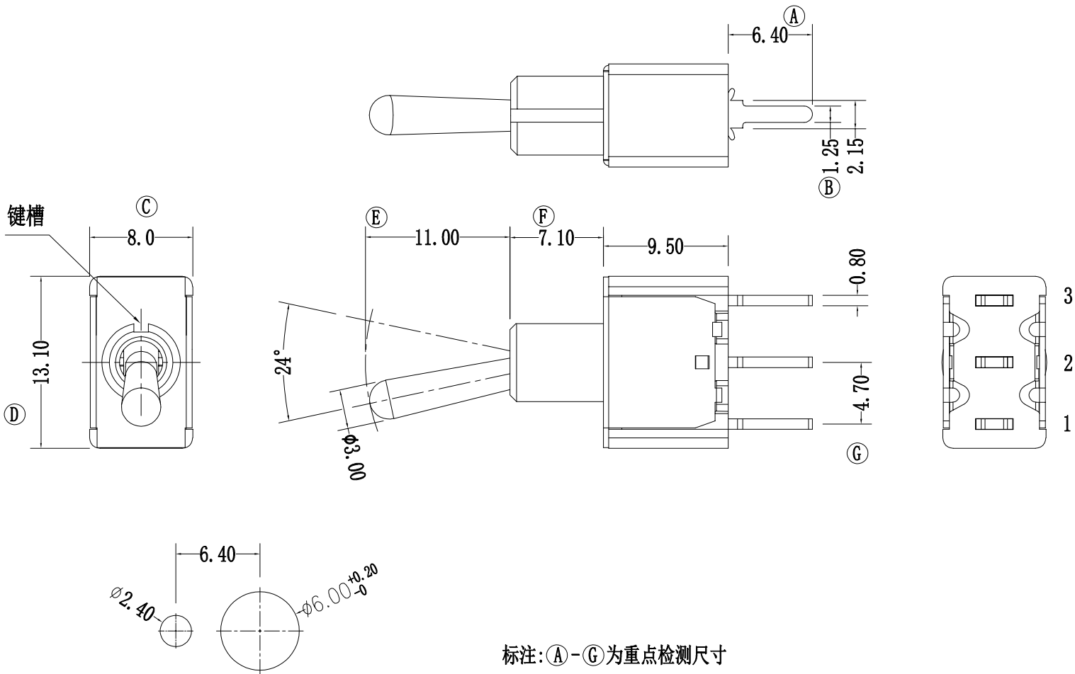
安装孔尺寸
