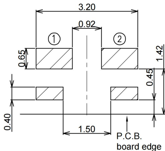
P.C.B. Layout(Tolerances ±0.05mm)
